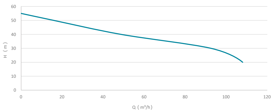
ZDP100-92/2 HCEV
